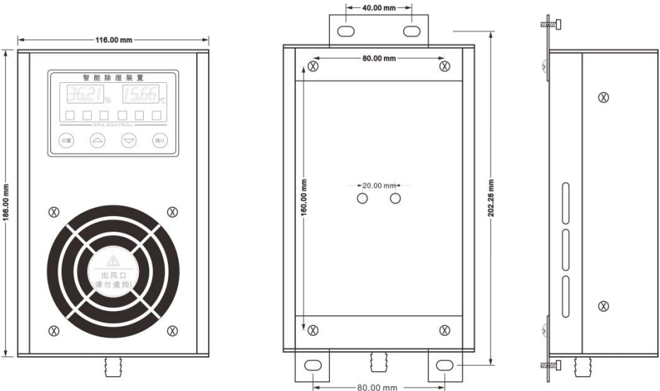
尺 寸 图
