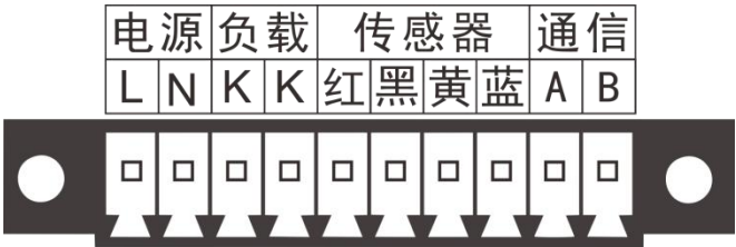
接 线 图
