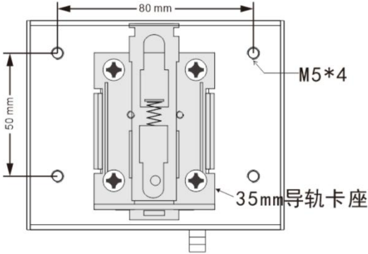
尺 寸 图
