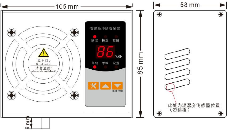
尺 寸 图
