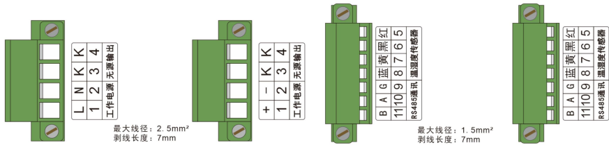
接线图
