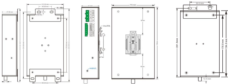
(1) “支架 1” 安装图
